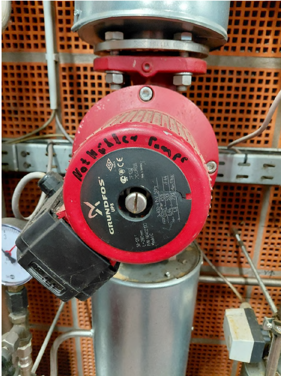
Abbildung 9: Notkühler Pumpe
