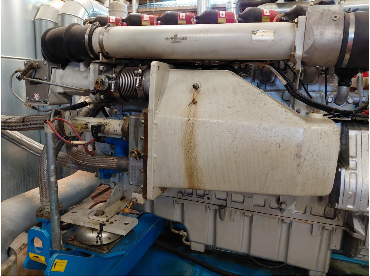
Abbildung 7: Gemischkühler
