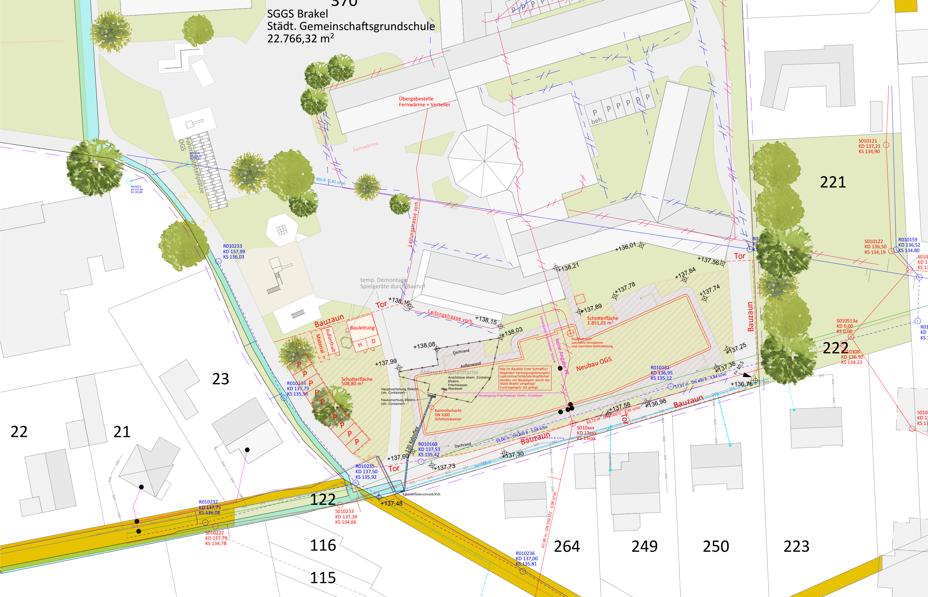
ANLAGE ZUR AUSSCHREIBUNG BAUSTELLENEINRICHTUNGSPLAN M 1:500 NEUBAU FÜR OGS-AUSBAU DER STÄDTISCHEN GEMEINSCHAFTSSCHULE BRAKEL
