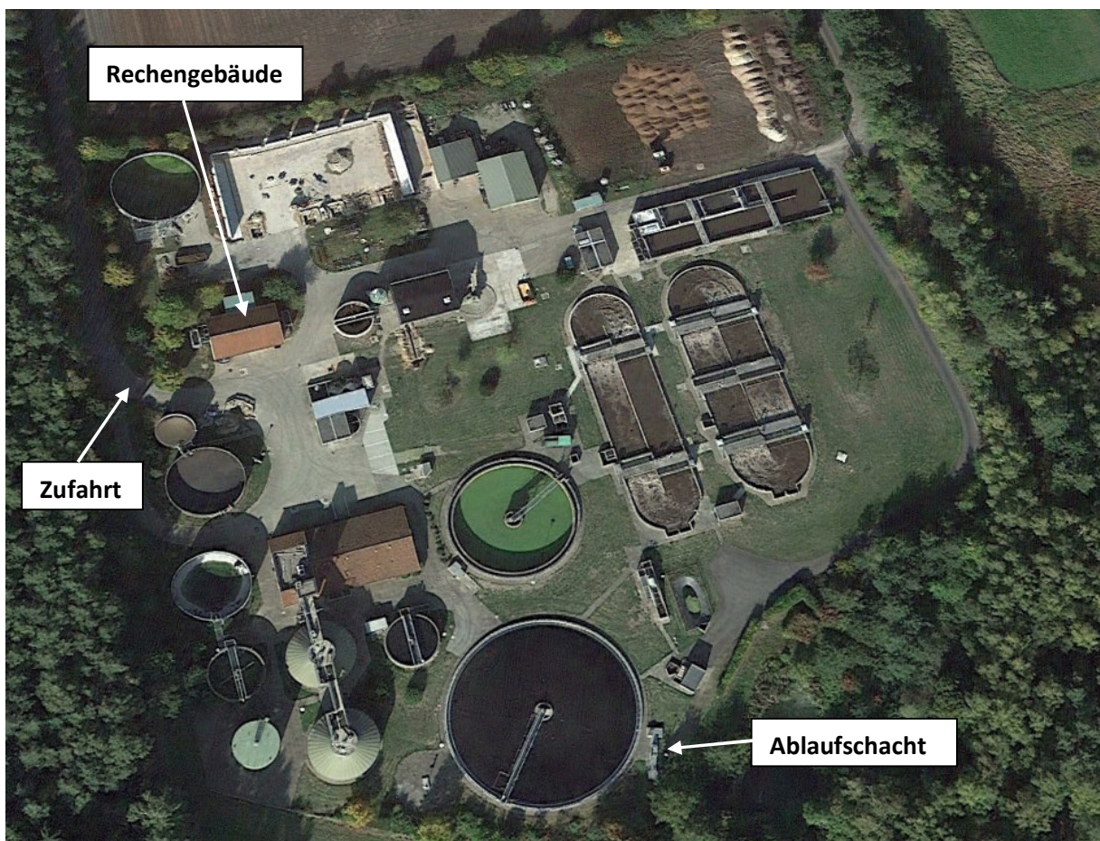
Kläranlage Soltau: Luftbild
