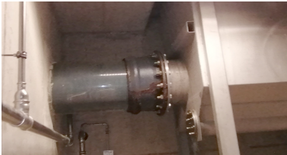
EG Rechengebäude: Ablauf Sandfang Straße 1
