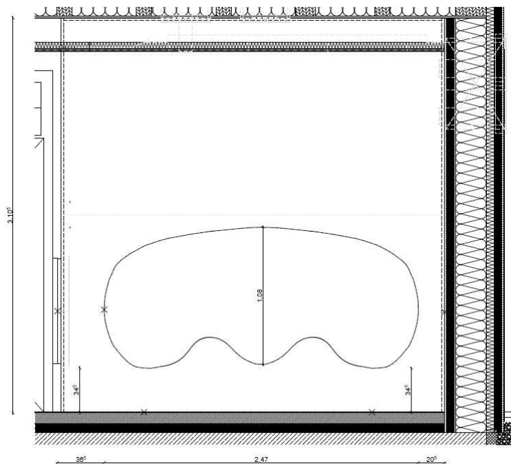
Schnitt a1
