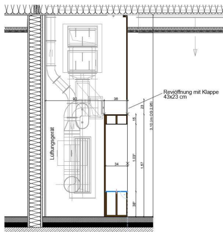
Schnitt a1
