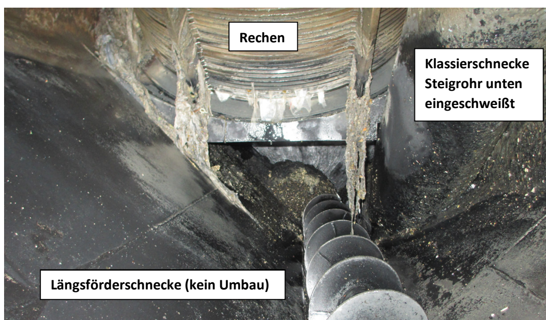
Bestand: Sandfang
