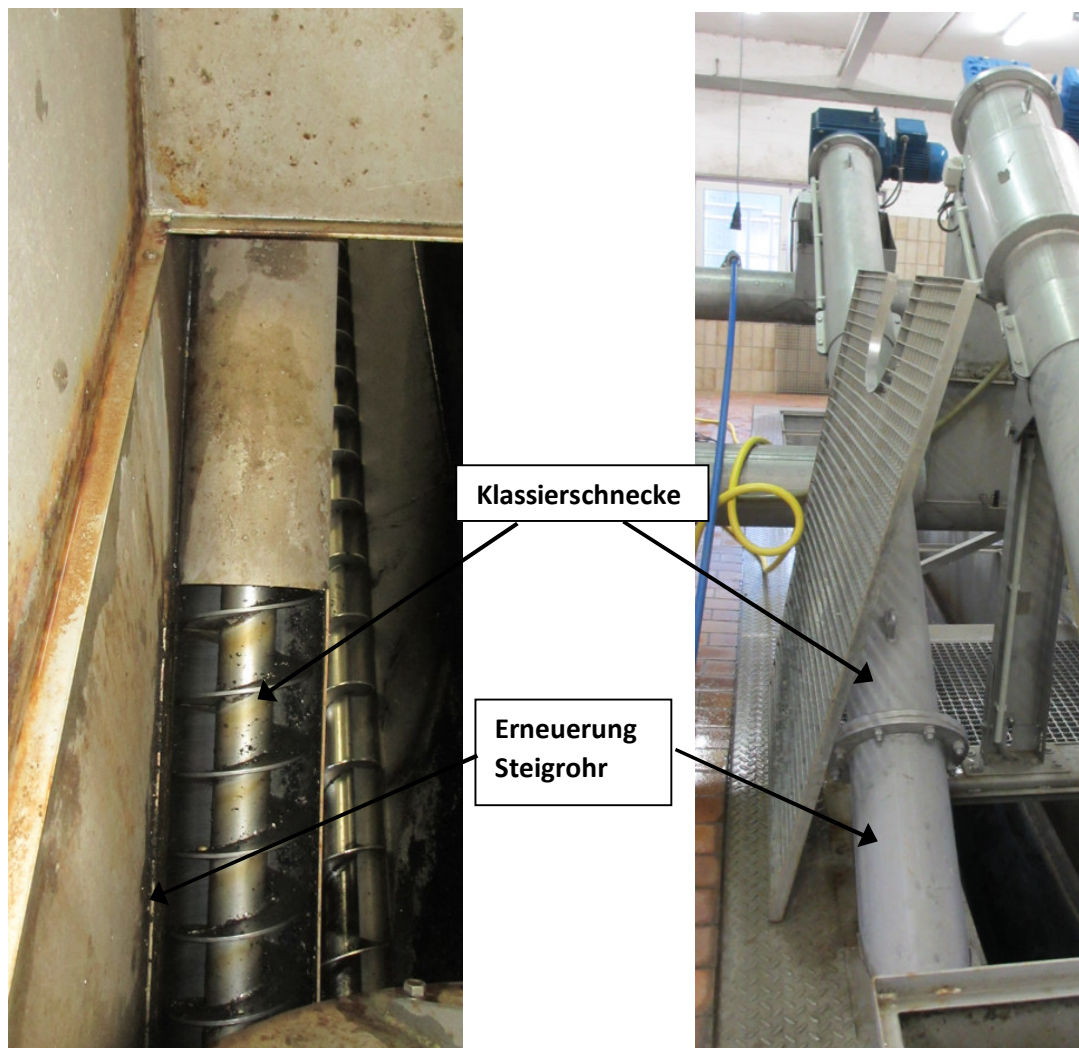
Bestand: Klassierschnecke
