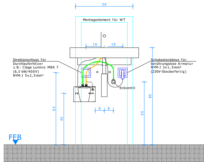
Detail Anschlüsse Waschtisch (M 1:20)
