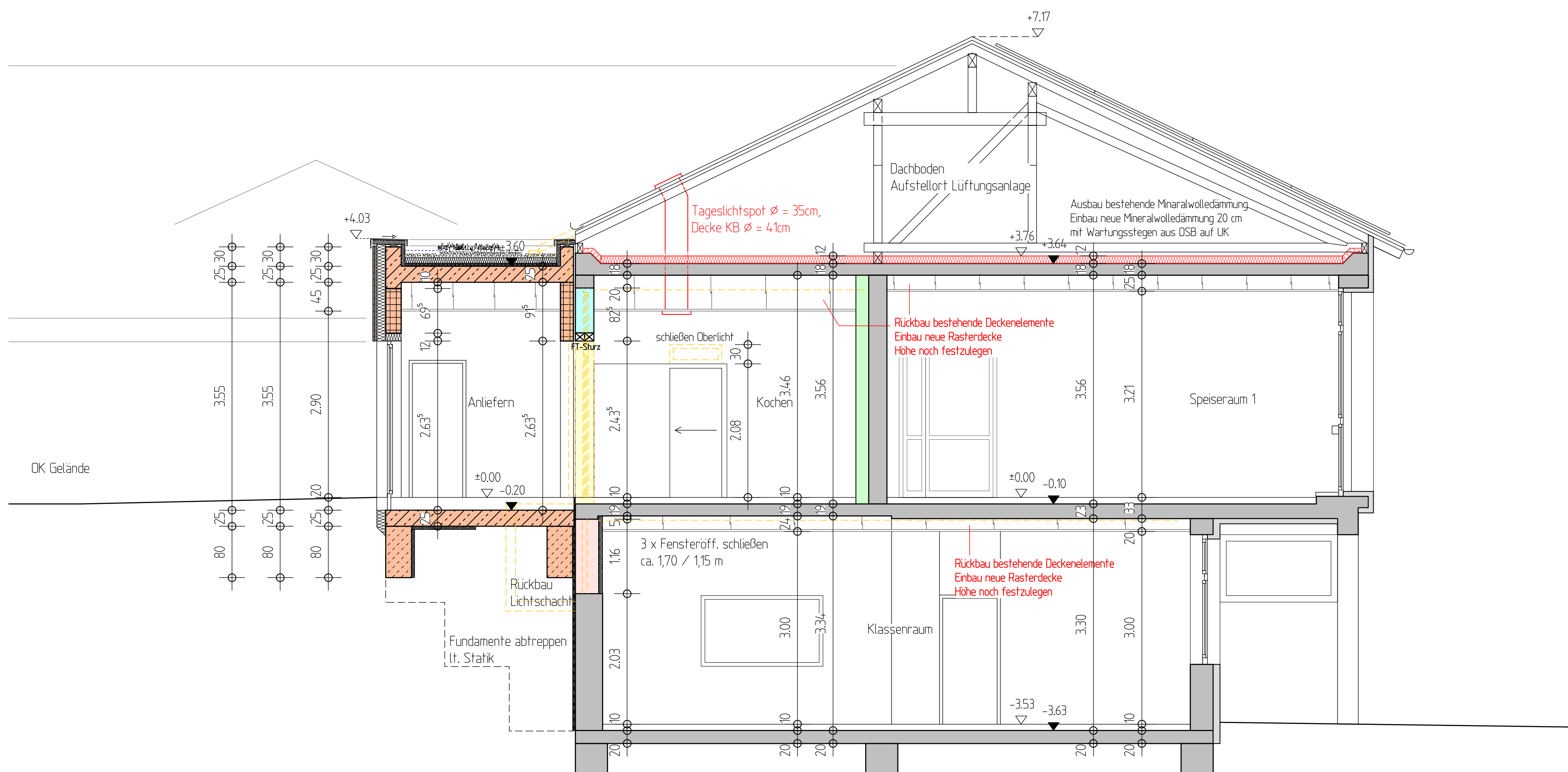
Schnitt B-B
