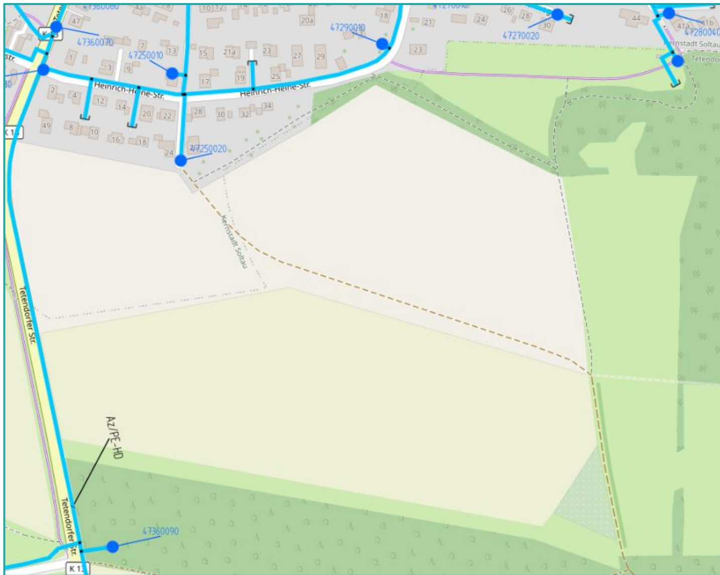
Abbildung 1: Hydranten (blaue Punkte) in der Umgebung des Neubaugebiets Tetendorfer Straße
